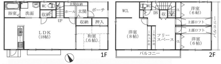
【間取り図】
